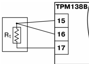
Рисунок 3.2 – Схема подключения ТС
