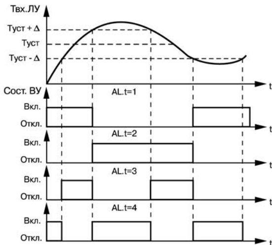
Рисунок 3.8 – Выходные характеристики компараторов
