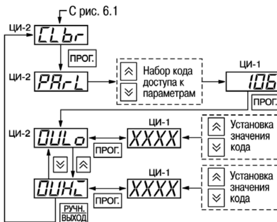
Рисунок Д.8 – Схема проведения юстировки ЦАП
