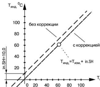
Рисунок 3.6 – Коррекция «Сдвиг характеристики»
