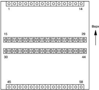
Рис. Б.1. Схема расположения контактов на приборе
