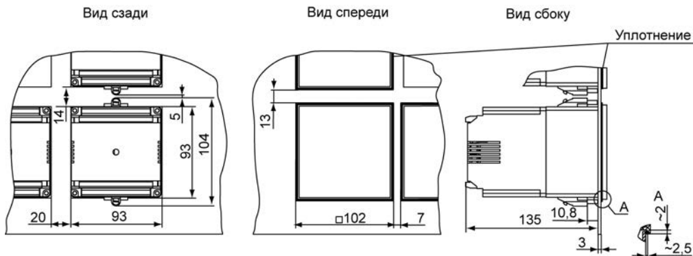
Рисунок А.2 – Габаритный чертеж TPM138B, установленного в щит толщиной 3 мм
