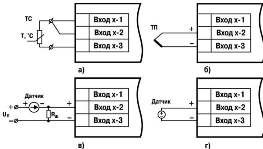
Рисунок Б.7 - Схемы подключения измерительных датчиков:
